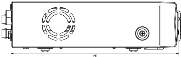
【側面図】
