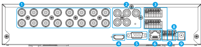
【背面図】
