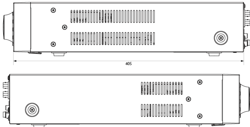
【側面図】
