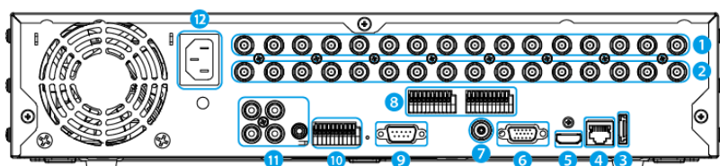
【背面図】
